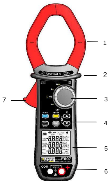
Figure 1 : la pince multimètre F607
