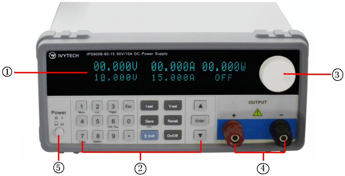
前面板图
