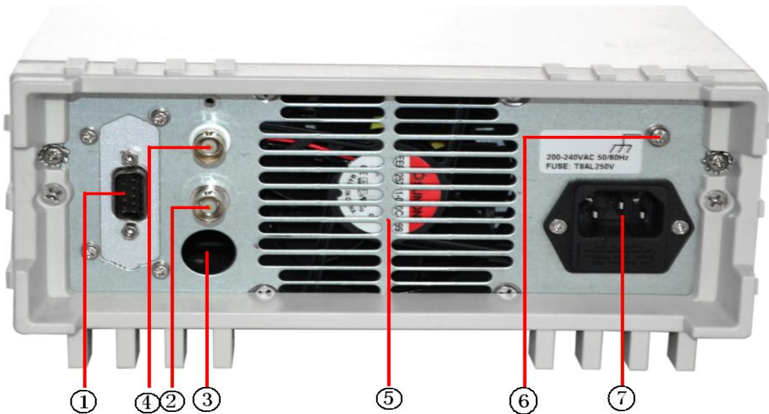
后面板图
