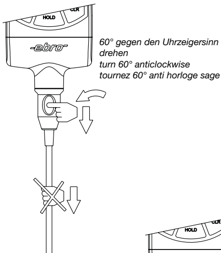
Fühler-Steckverbindung Plug-in connector Connecteur embrochable
