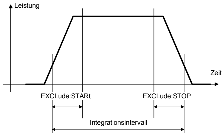
Abbildung 6-9: Wirkung der Befehle SENS[1..4]:TIM:EXCL:STAR und :STOP
