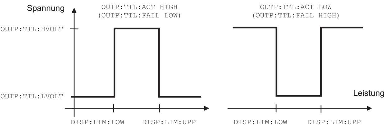
Abbildung 6-6: Spannung am TTL-Ausgang
