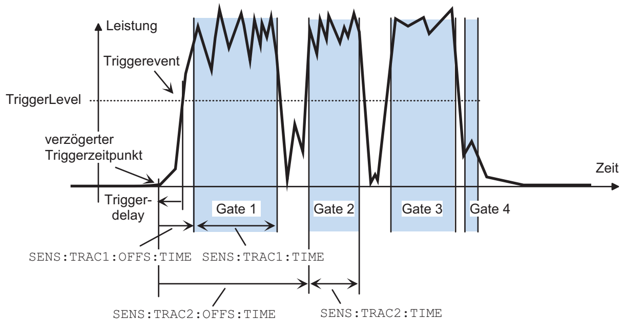
Abbildung 6-8: Timingparameter für den Timegate-Modus.
