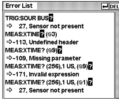
Bild 4-46 Errorlist – Dialog
