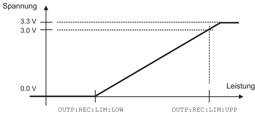
Abbildung 6-5: Kennlinie der Analogausgänge
