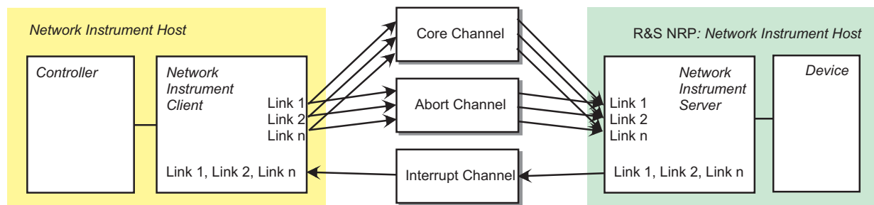
Diagramm einer VXI11-Verbindung mit mehreren Links
