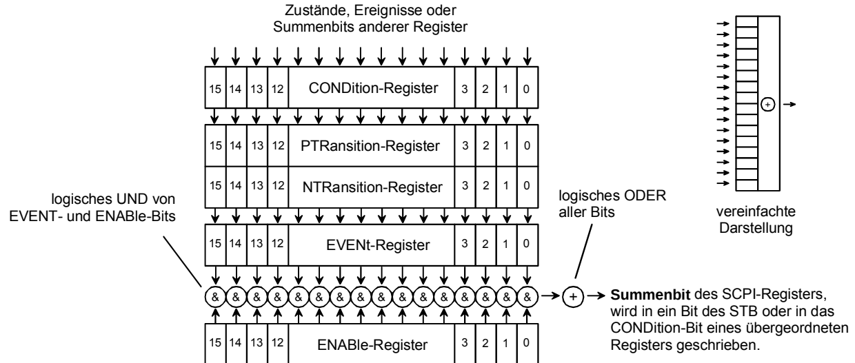
Abbildung 6-10: Standard SCPI-Statusregister
