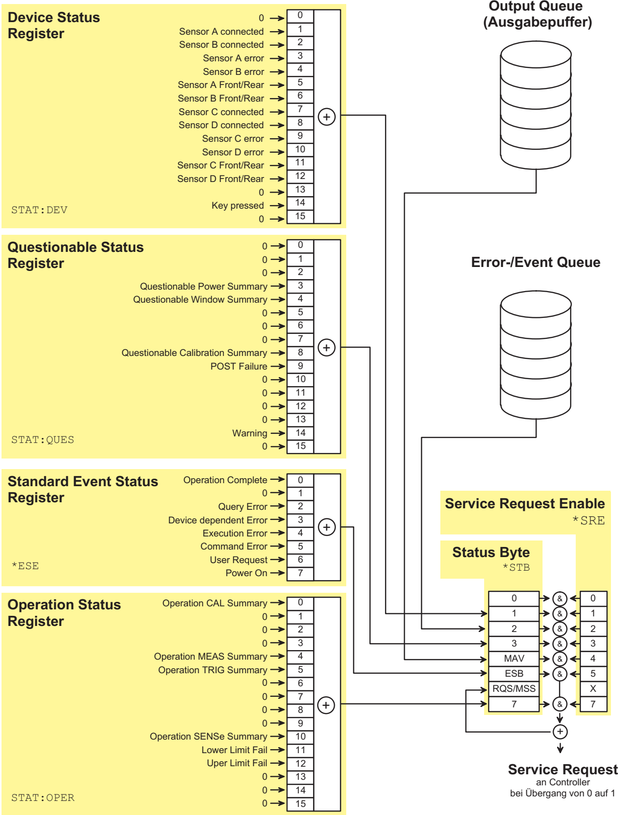
Abbildung 6-11: Überblick über den Aufbau des Status Reporting Systems
