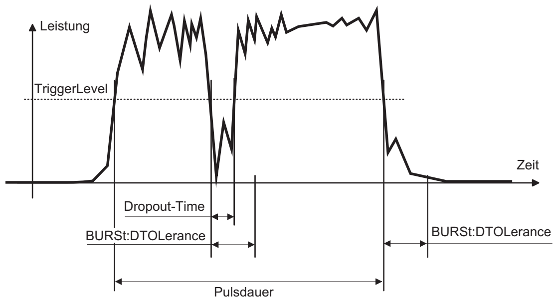
Abbildung 6-7: Zur Bedeutung der Dropout-TOLerance.
