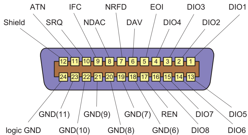
Abbildung 6-14: Pinbelegungen der IEC-Bus-Schnittstelle
