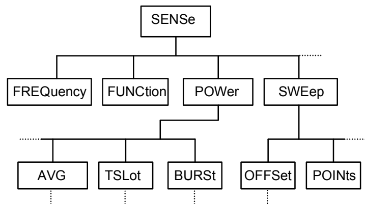
Abbildung 5-1: SCPI-Befehlsbaum
