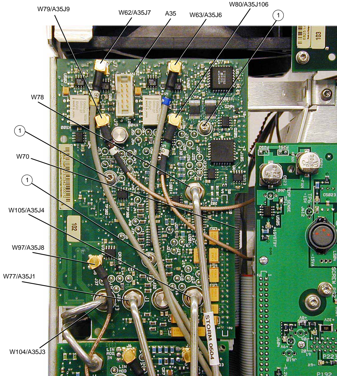
Figure 3-60 A35 3–20 GHz I/Q MOD
