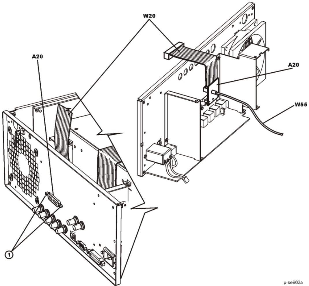
Figure 3-25 A20 SMI
