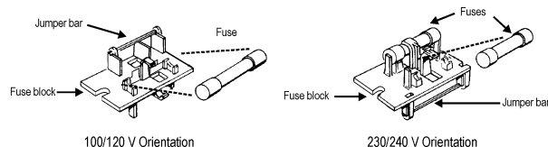
Figure 6. Orientation du bloc de fusibles pour le fonctionnement à 100/120 V c.a. et à 230/240 V c.a.
