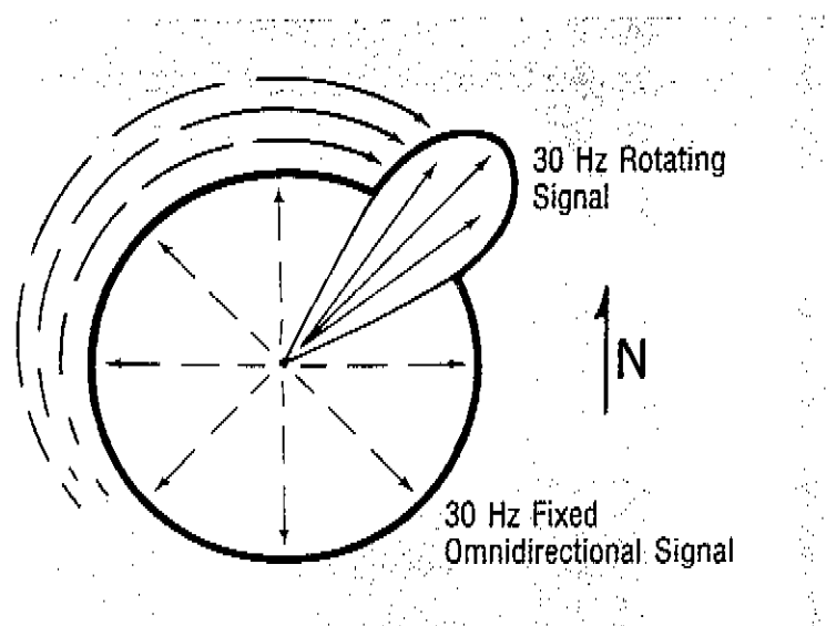
VOR Antenna Pattern
