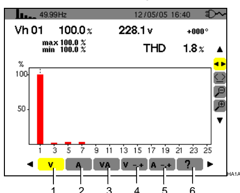
Figure 34 : Exemple d'affichage des Harmoniques.
