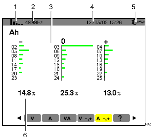
Figure 40 : Exemple d'affichage des harmoniques de courant en fonction de leur effet.
