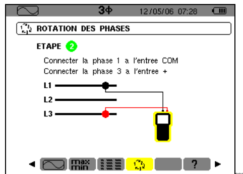
Figure 24 : L'étape n° 2 de Rotation des phases.
