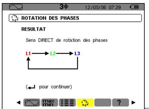
Figure 27 : Exemple du résultat d'une mesure d'un sens de phases direct.
