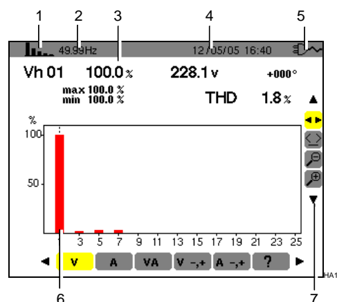
Figure 36 : Exemple d'affichage des harmoniques de la tension.
