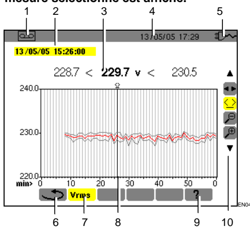
Figure 52 : Exemple d'écran d'enregistrement de mesure.
