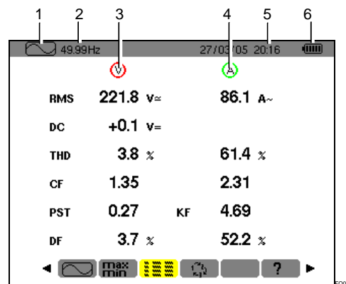
Figure 21 : Les informations de l'écran d'Affichage simultané.
