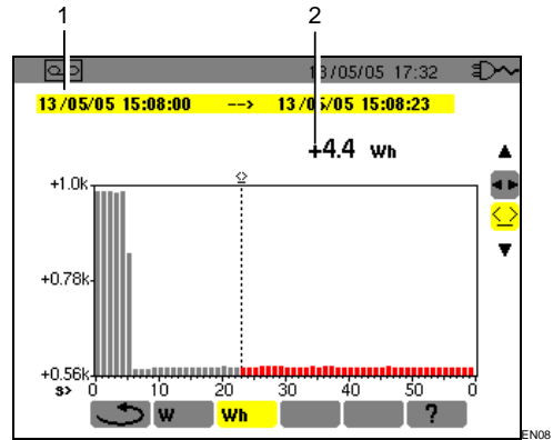
Figure 56 : Exemple d'écran de mesure d'énergie.
