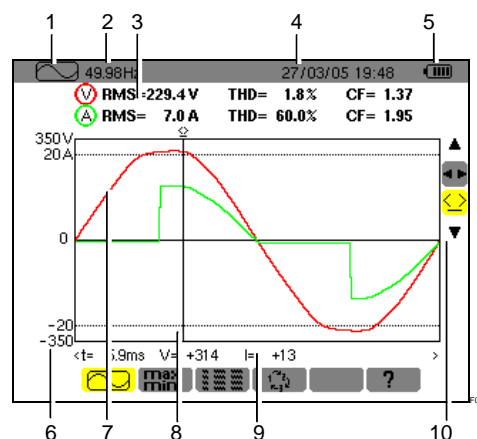
Figure 19 : Les informations de l'écran Formes d'ondes.
