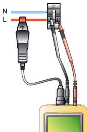
Figure 69 : Connexion en monophasé. 005
