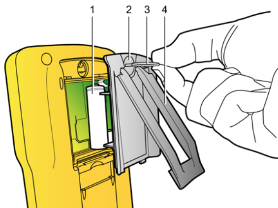
Figure 4 : Accès aux accumulateurs. 003
