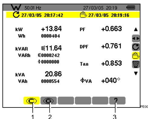
Figure 30 : Exemple d'affichage de mesures de Puissances et énergies.
