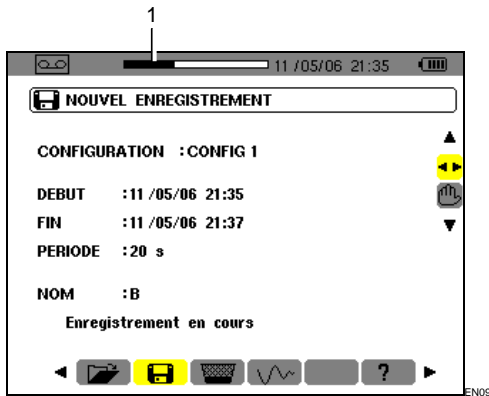
Figure 49 : La bande noire indique le temps écoulé par rapport au temps total de l'enregistrement en cours.
