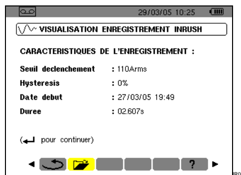
Figure 61 : Rappel des spécifications de l'enregistrement Inrush .
