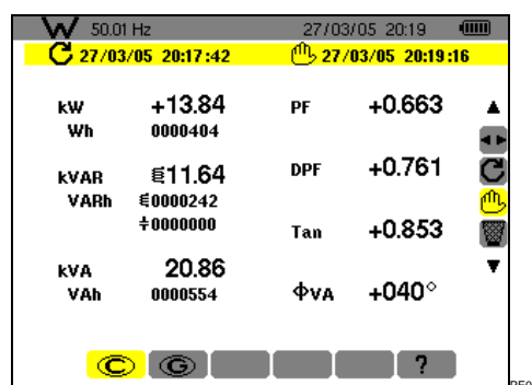
Figure 32 : Exemple d'affichage de mesures de puissances et d'énergies après un comptage.
