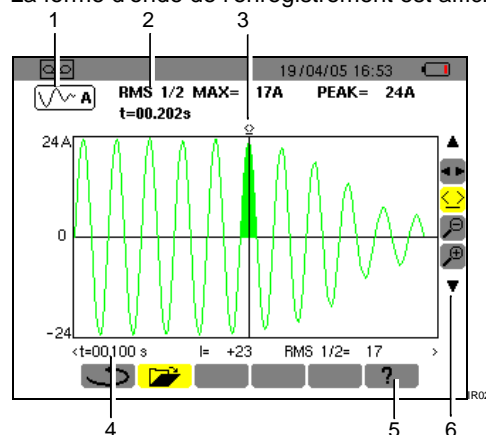
Figure 62 : Visualisation d'une forme d'onde.
