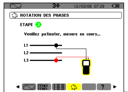
Figure 25 : La mesure est en cours.
