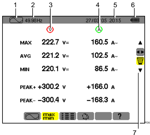
Figure 20 : Les informations de l'écran Max-Min.
