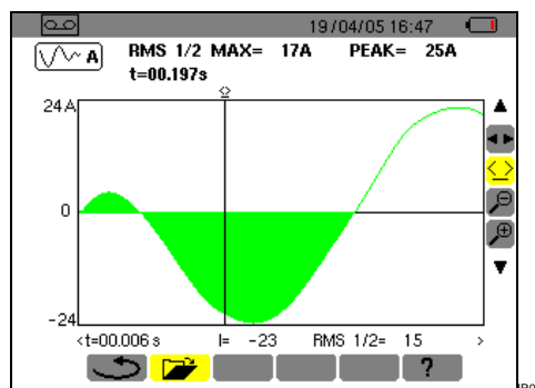
Figure 64 : Zoom maximal d'une partie d'une forme d'onde.
