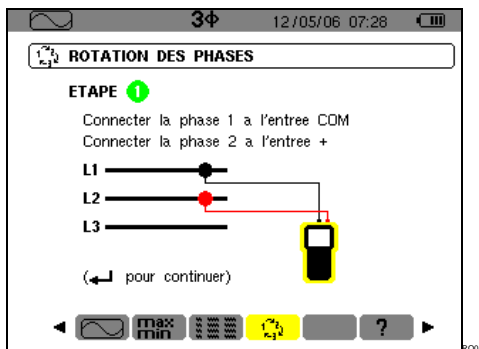
Figure 22 : L'étape n° 1 de Rotation des phases.
