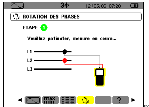
Figure 23 : L'écran lors de la mesure.
