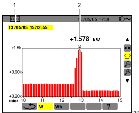
Figure 55 : Exemple d'écran de mesure de puissance active.
