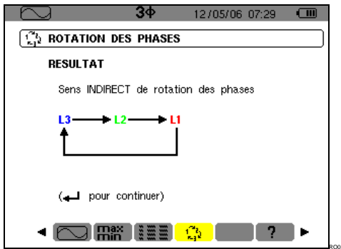
Figure 26 : Exemple du résultat d'une mesure d'un sens de phases indirect.
