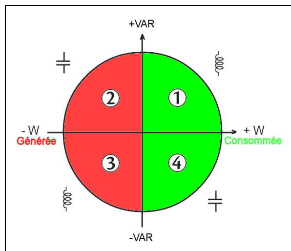
Figure 73 : La représentation des quatre quadrants de puissance. 010
