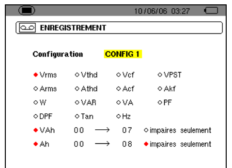
Figure 13 : Dans cet exemple (ligne du bas), les harmoniques 0 à 7 seront enregistrées pour la mesure du VAh. Pour la mesure des Ah, seules les harmoniques impaires comprises entre 0 et 8 (c'est-à-dire 1, 3, 5 et 7) seront enregistrées.
