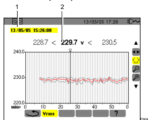
Figure 53 : Exemple d'écran de mesure Vrms.
