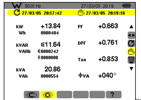
Figure 33 : Exemple d'affichage de mesures de puissances et d'énergies après un comptage.
