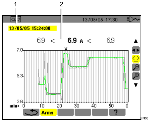
Figure 54 : Exemple d'écran de mesure Arms.
