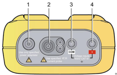
Figure 68 : Les connecteurs en partie supérieure.
