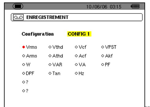
Figure 11 : Dans cet exemple, seules les mesures relatives à la Vrms seront enregistrées.
