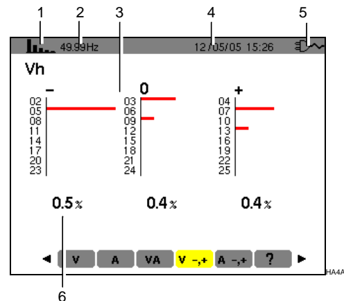
Figure 39 : Exemple d'affichage des harmoniques de tension en fonction de leur effet.
