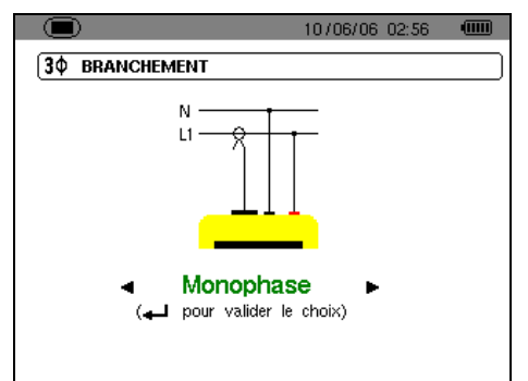
Figure 9 : Le menu Branchement.
