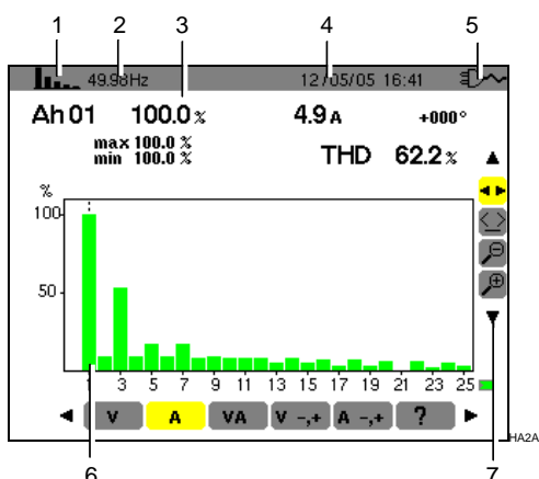
Figure 37 : Exemple d'affichage des harmoniques du courant.
