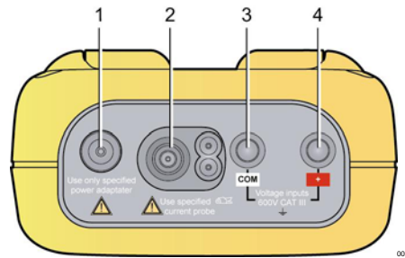
Figure 3 : Les bornes en partie supérieure.
