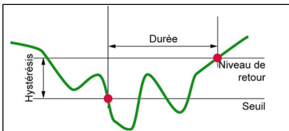
Figure 72 : L'hystérésis pour une détection de sous-tension. 009
