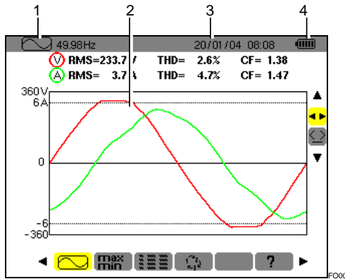
Figure 2 : Exemple d'un écran de visualisation.
