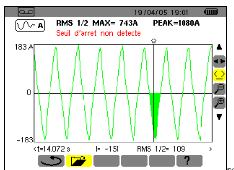
Figure 63 : Un message est affiché lorsque le seuil n'a pas été détecté.
