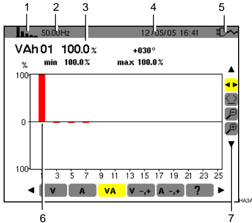
Figure 38 : Exemple d'affichage des harmoniques de la puissance apparente.
