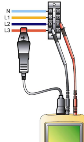
Figure 70 : Connexion en triphasé équilibré. 006
