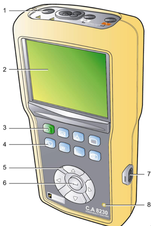
Figure 1 : Vue générale du C.A 8230.
