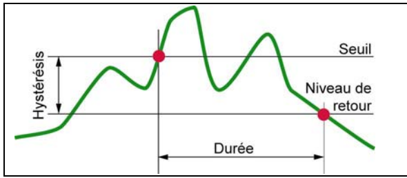
Figure 71 : L'hystérésis pour une détection de sous-tension. 008
