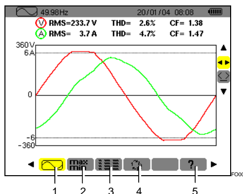
Figure 17 : Exemple d'affichage de Formes d'ondes.
