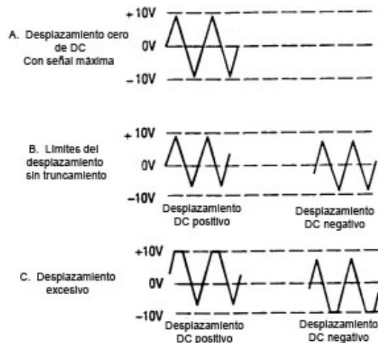
Figura 3. Uso del control DC OFFSET
