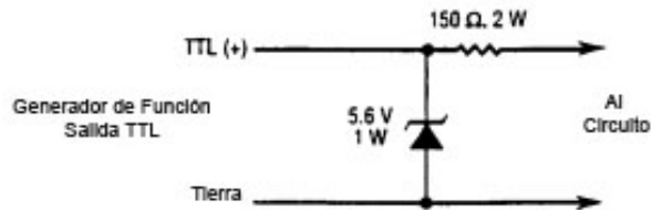
Figura 5. Circuito de protección para la salida TTL
