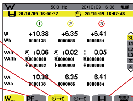
Figure 78 : l'écran du mode puissances et énergies
