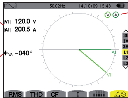
Figure 65 : l'écran d'affichage du diagramme de Fresnel en L1
