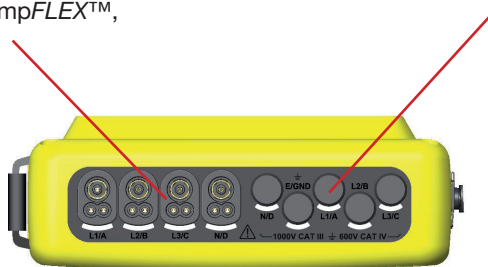
Figure 3 : les connecteurs en partie supérieure
