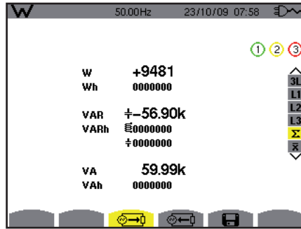
Figure 82 : l'écran d'affichage des sommes des énergies consommées
