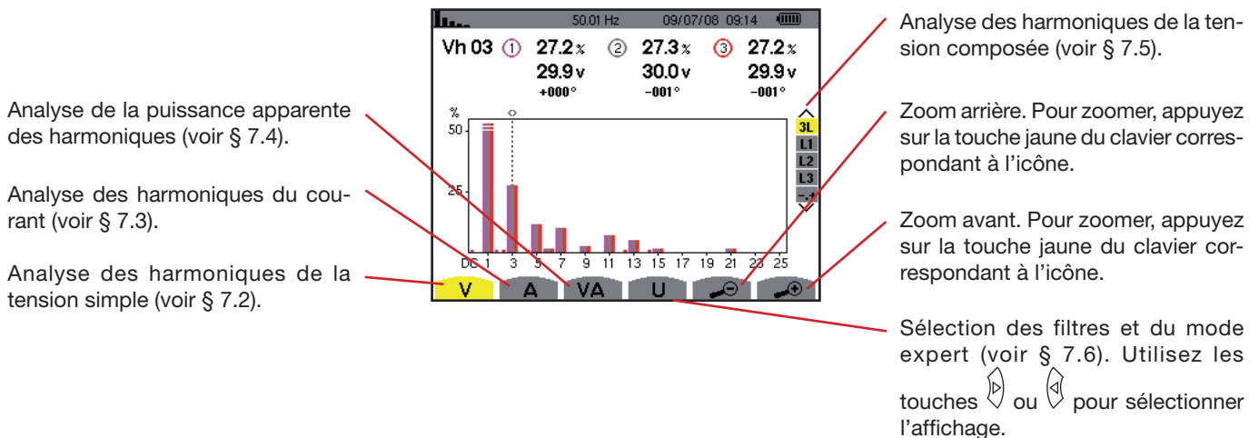
Figure 33 : l'écran du mode harmonique
