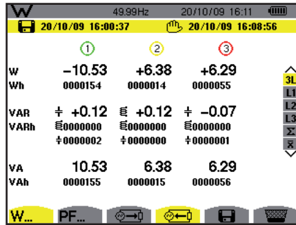
Figure 84 : l'écran d'affichage énergies générées pour les 3 phases (3L)
