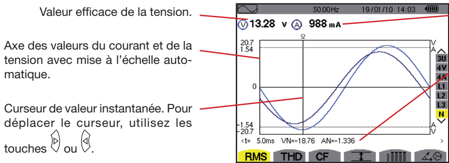
Figure 48 : l'écran d'affichage RMS pour le neutre
