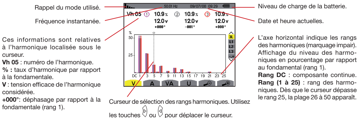
Figure 34 : exemple d'affichage des harmoniques de la tension simple (harmonique n° 5 : Vh05) en 3L
