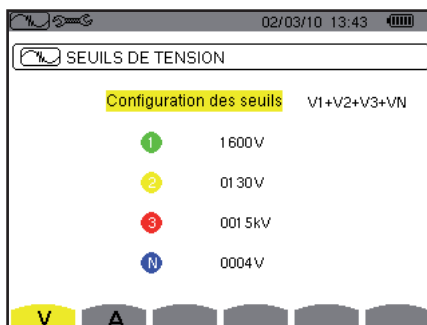
Figure 15: l'écran Seuils de tension dans le menu Mode transitoire
