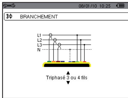
Figure 96 : connexion en triphasé 3 ou 4 fils
