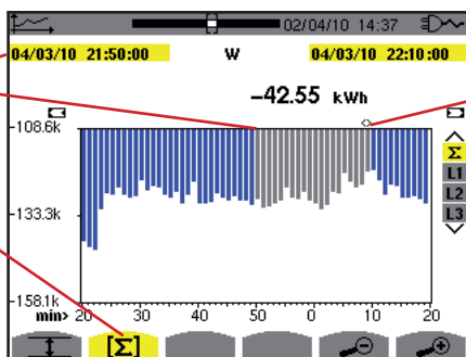
Figure 110 : Wh ( \Sigma ) sans MIN-AVG-MAX
