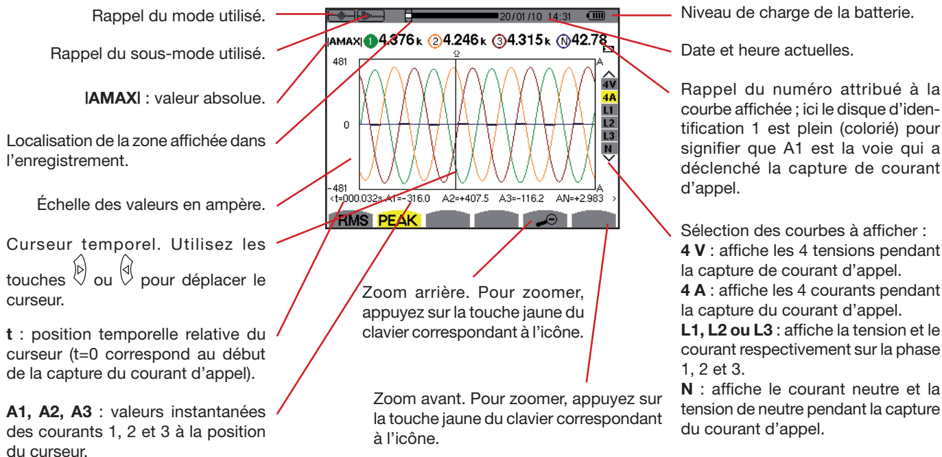
Figure 31 : l'écran d'affichage PEAK en 4A
