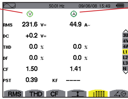
Figure 63 : L'écran affichage simultané en L1
