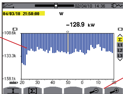
Figure 108 : W ( \Sigma ) sans MIN-AVG-MAX
