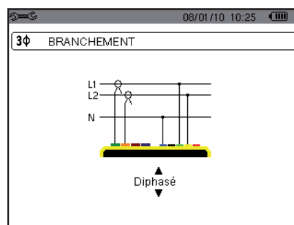
Figure 95 : connexion en diphasé
