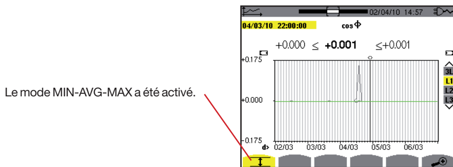
Figure 113 : \cos \Phi (L1) avec MIN-AVG-MAX
