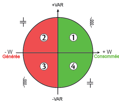
Figure 98 : diagramme des 4 quadrants
