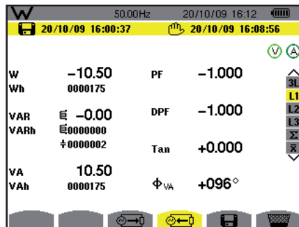
Figure 85 : l'écran d'affichage énergies générées pour la phase 1 (L1)
