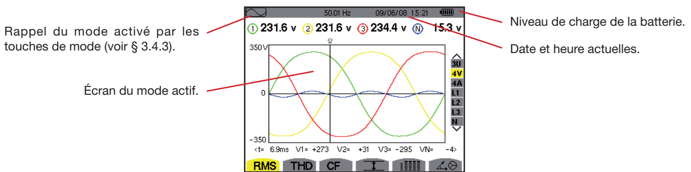
Figure 2 : exemple d'un écran de visualisation
