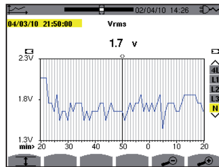
Figure 102 : Vrms (N) sans MIN-AVG-MAX
