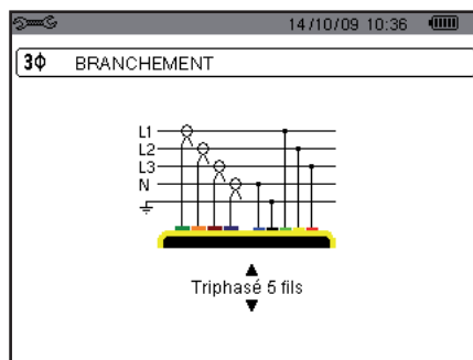
Figure 11 : le menu Branchement
