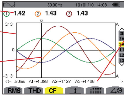
Figure 54 : l'écran d'affichage CF en 3A
