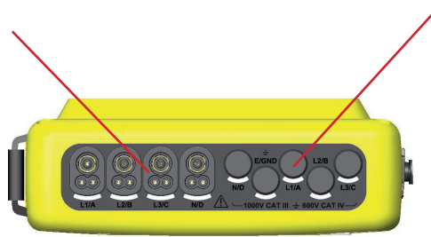
Figure 93 : les connecteurs en partie supérieure
