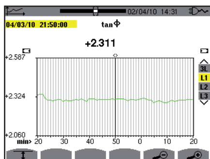
Figure 106 : tan Φ (L1) sans MIN-AVG-MAX
