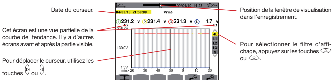
Figure 100 : Vrms (4L) sans MIN-AVG-MAX
