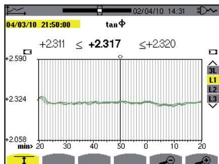
Figure 107 : tan Φ (L1) avec MIN-AVG-MAX
