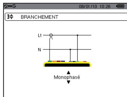
Figure 94 : connexion en monophasé
