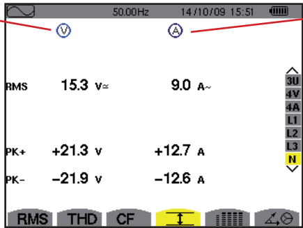
Figure 59 : l'écran d'affichage Max-Min du neutre
