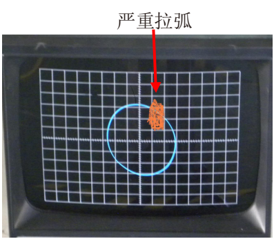
图三：严重拉弧的李沙育图形
