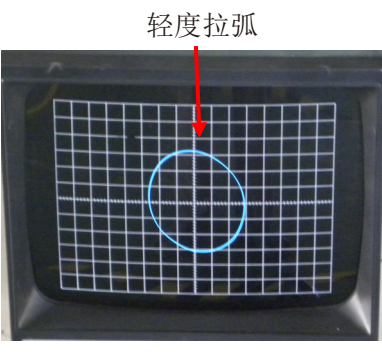
图二：轻度拉弧的李沙育图形
