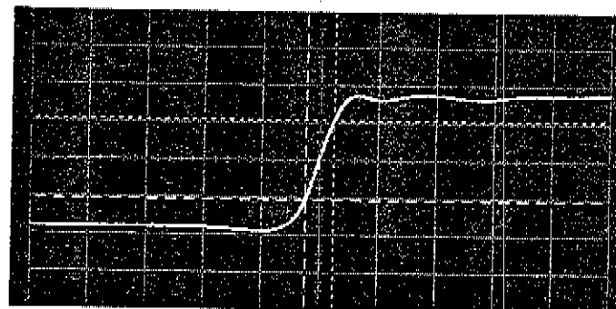
Figure 6-6. TRIGGER Risettime - 100 ps/div
