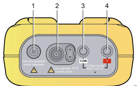
Figura 68: los conectores en la parte superior.
