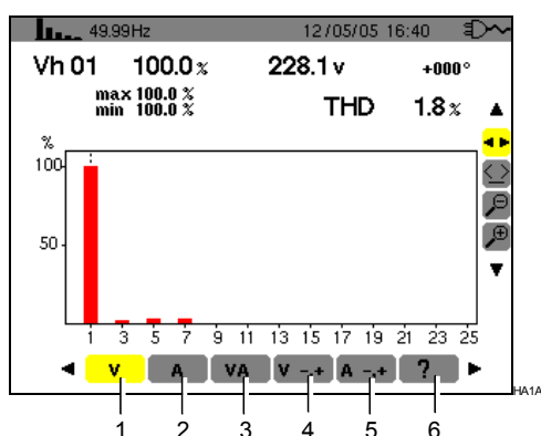
Figura 34: ejemplo de visualización de los Armónicos.
