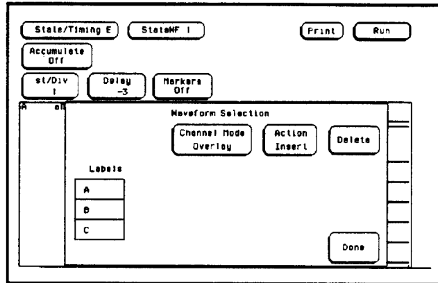
Figure 10-6. Action Insert/Replace
