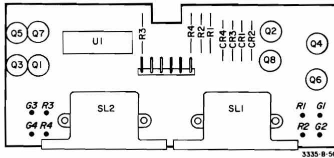
A25 -hp- Part No. 5060-9597
