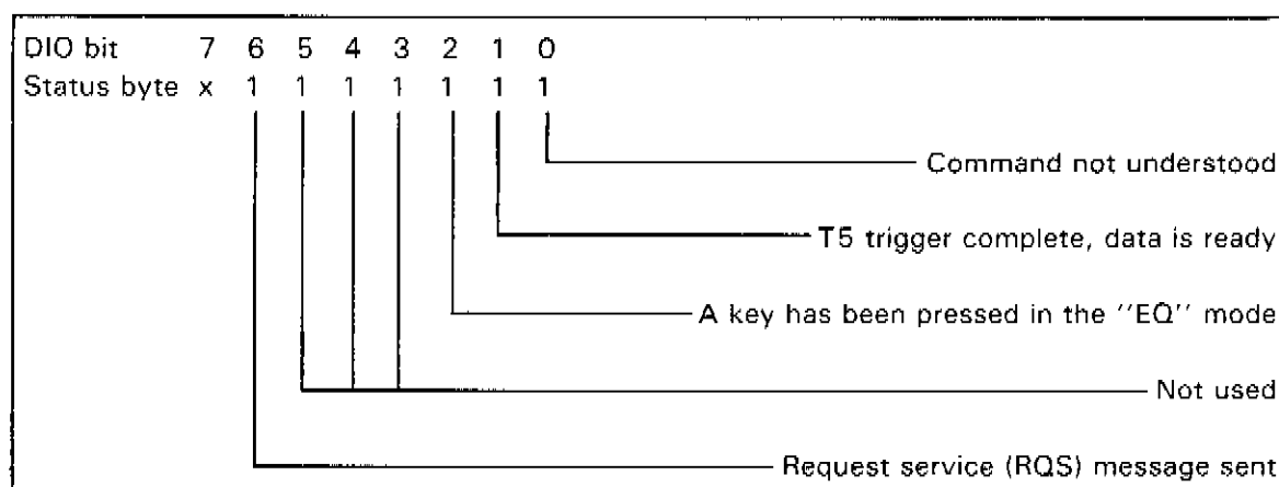
Figure 3-2-4. Status Byte.
