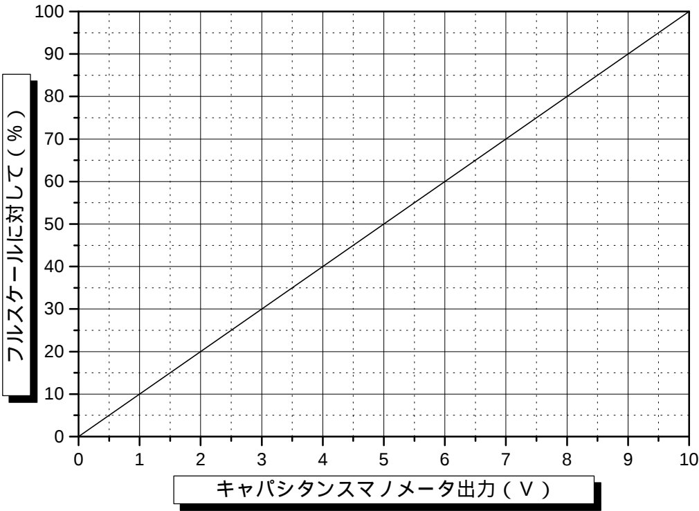
図 1. キャパシタンスマノメータ出力信号グラフ
