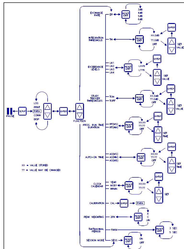
Figure 11. Parameter Setup Menu
