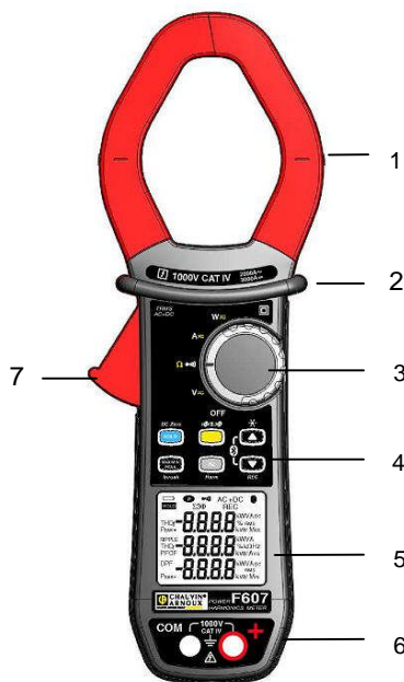
Figura 1 : la pinza multimétrica F607
