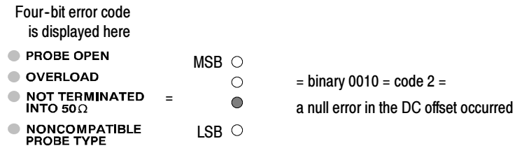
Figure 3- 16: Interpreting the error code display
