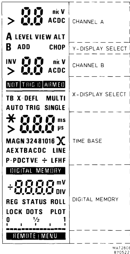
Abb. 3.2 Flüssigkristall-Anzeige (LCD)
