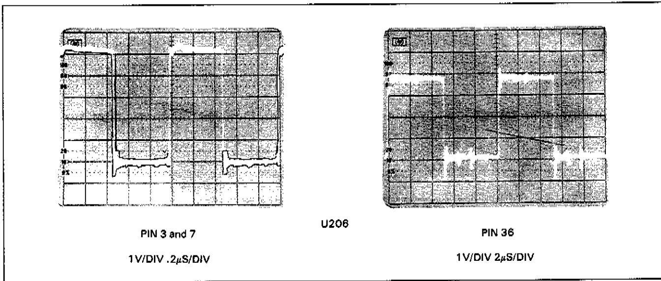
Figure 8-6. SA Clocks
