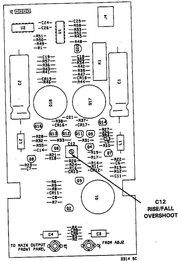
A5 03314-66505 X3 OUTPUT
