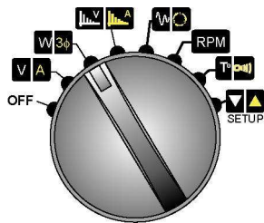
Figure 17 : Le commutateur rotatif en position W3Φ .
