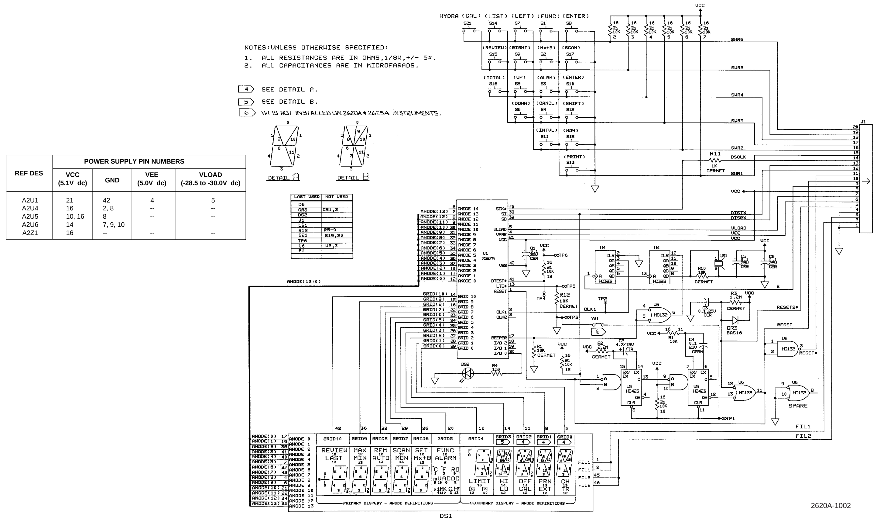
Figure 8-3. A2 Display PCA (cont)
