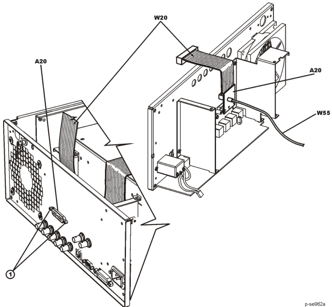
Figure 3-26 A20 SMI
